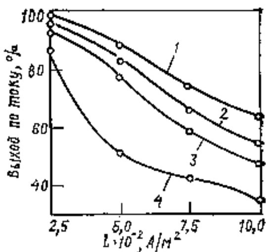
Рис. 3.4. Влияние плотности тока на выход цинка по току из цианидного электролита
