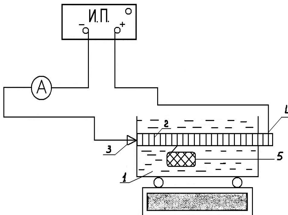
Рис. 4.3. Схема установки для электроосаждения лакокрасочных покрытий:
