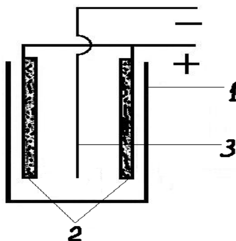
Рис. 4.1. Схема весового медного кулонометра:
