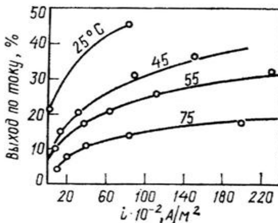
Рис. 3.15. Влияние катодной плотности тока и температуры на выход хрома по току в электролите, содержащем 250 \text{ г/л } CrO_3 и 2,5 \text{ г/л } H_2SO_4
