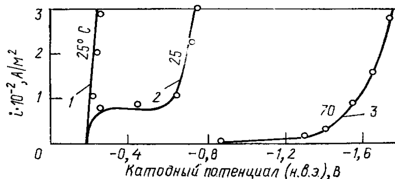
Рис. 3.5. Поляризационные кривые электроосаждения олова из кислых и щелочных электролитов при 25 °С:
