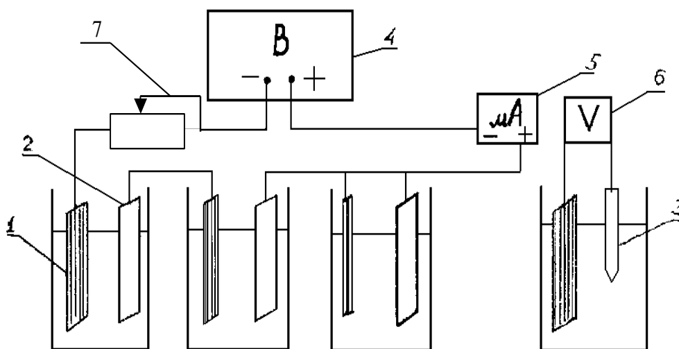
Рис. 4.4. Схема установки для исследования электрохимической защиты сталей от коррозии:
