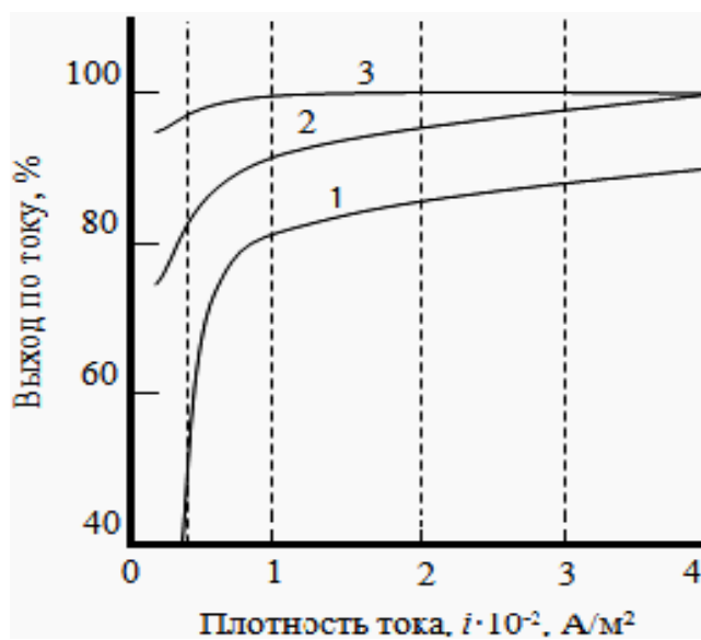
Рис. 3.12. Зависимость выхода никеля по току из электролита, содержащего 140 г/л NiSO 4 ·7H 2 O, 20 г/л NiCl 2 ·6H 2 O и 25 г/л H 3 BO 3 , от плотности тока Условия электролиза: 1 – рН = 1,9, 25 °С; 2 – рН = 1,9, 52 °С; 3 – рН = 5,3, 25 °С
