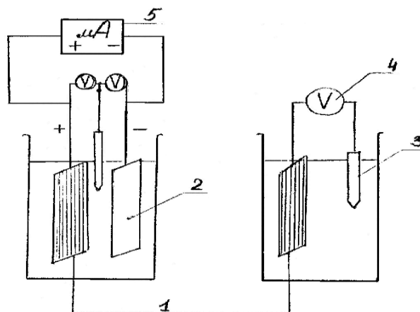
Рис. 4.5. Схема установки для исследования защиты стали от коррозии с помощью протектора: 1 – электрод; 2 – протектор; 3 – хлорсеребряный электрод; 4 – цифровой вольтметр; 5 – миллиамперметр
