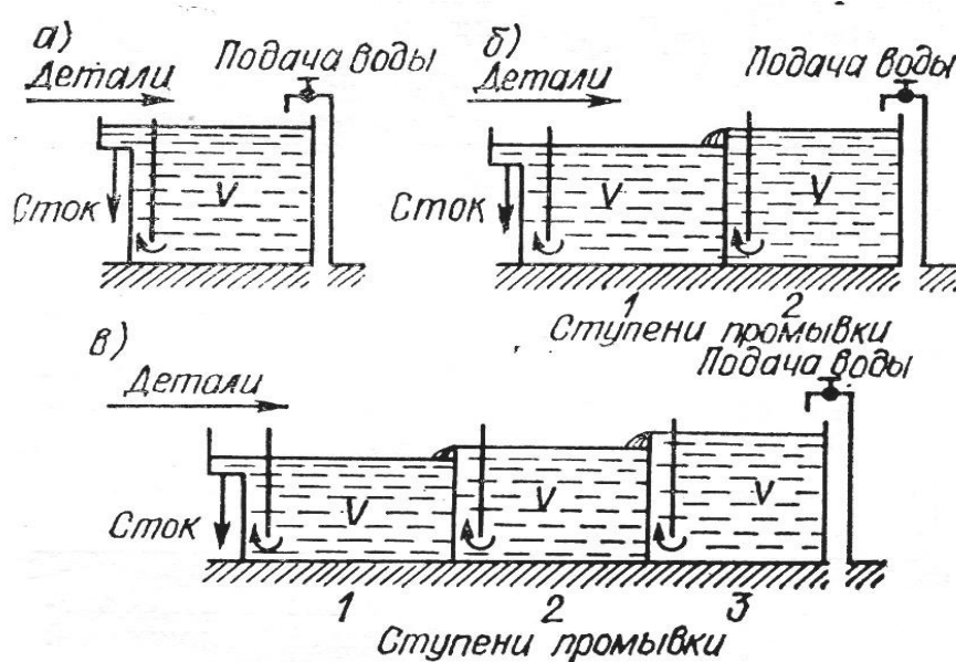
Рис. 3.1. Основные схемы промывки деталей:
