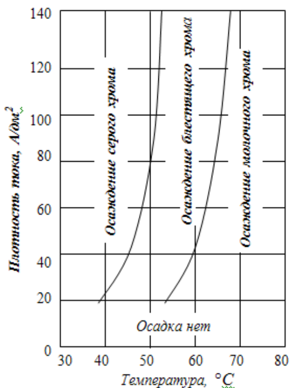
Рис. 3.17. Расположение зон различных хромовых осадков (CrO 3 – 250 г/л, H 2 SO 4 – 2,5 г/л)
