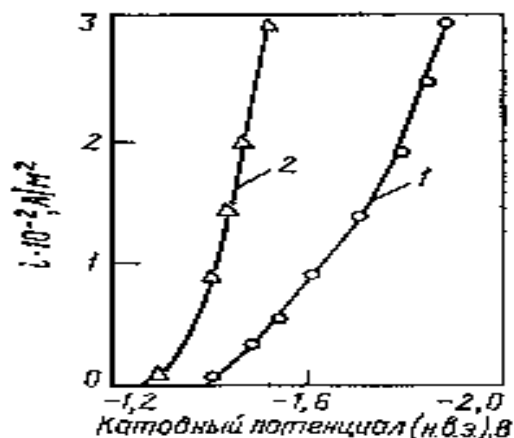
Рис. 3.3. Поляризационные кривые электроосаждения цинка из комплексных электролитов:
