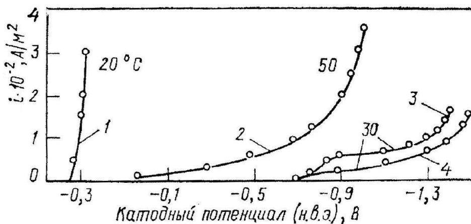
Рис. 3.9. Поляризационные кривые электроосаждения меди из различных электролитов:
