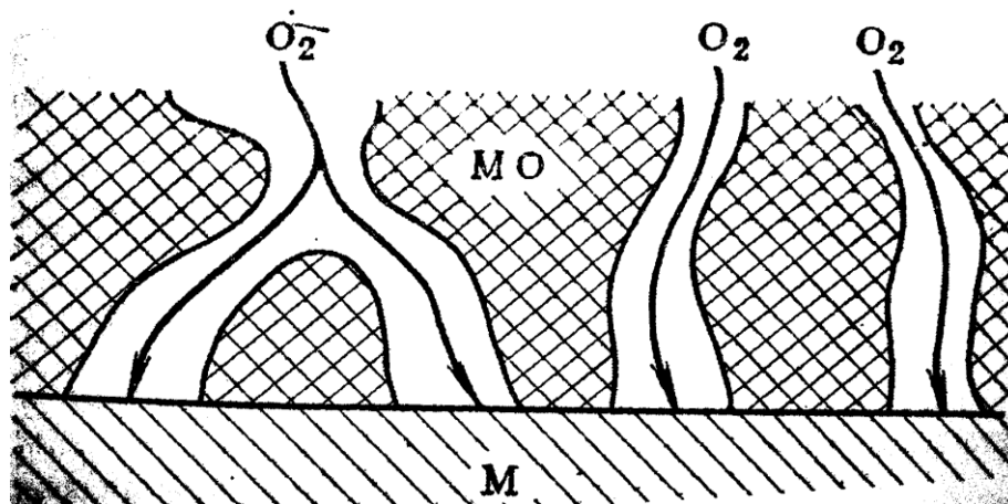
Рис. 1.7. Схема образования пористой оксидной пленки на поверхности металла
