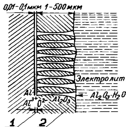
Рис. 3.18. Схема образования оксидной пленки на алюминии:
