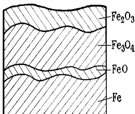
Рис. 1.11. Схема образования окалины при нагревании железа на воздухе
