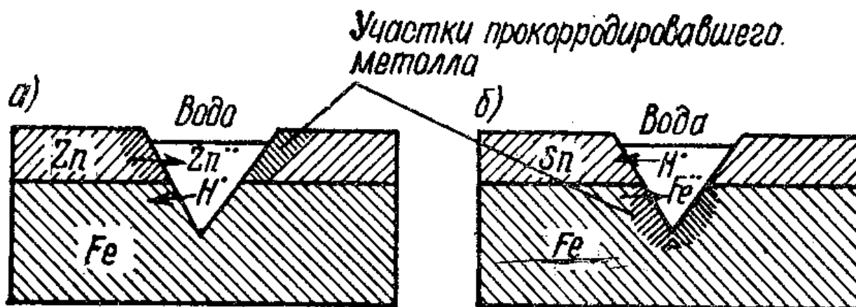
Рис. 2.1. Схема коррозии железа:
