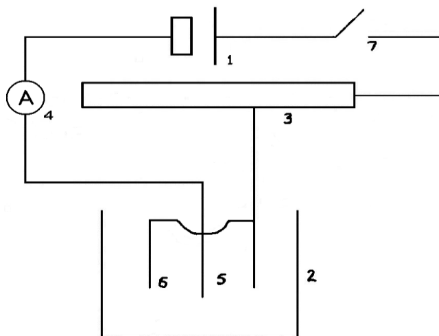
Рис. 4.2. Схема питания электролизера током:
