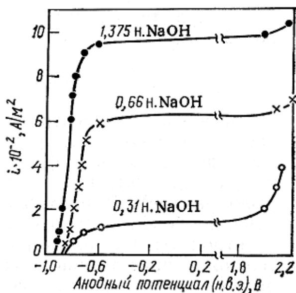
Рис. 3.7. Влияние концентрации свободной щелочи в станнатном электролите на зависимость анодного потенциала плотности тока (температура электролита 70 °С)
