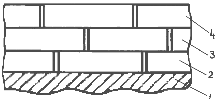
Рис. 3.8. Пористость в многослойном покрытии: 1 – основа – сталь; 2 – матовое никелевое покрытие; 3 – медное покрытие; 4 – блестящее никелевое покрытие
