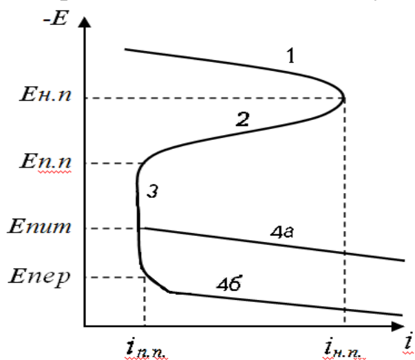
Рис. 1.6. Потенциостатическая анодная поляризационная кривая: 1 – область активного растворения металла; 2 – активно-пассивное состояние металла; 3 – пассивное состояние металла; 4 – нарушение пассивного состояния металла; а – питтингообразование; б – перепассивация; E_{н.п.} и i_{н.п.} – потенциал и ток начала пассивации; E_{п.п.} и i_{п.п.} – потенциал и ток полной пассивации; E_{пит} – потенциал питтингообразования; E_{пер} – потенциал перепассивации
