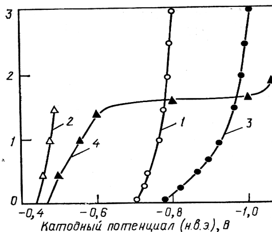
Рис. 3.2. Поляризационные кривые электроосаждения цинка и кадмия из кислых электролитов: 1 – 215 г/л ZnSO_4 , 30 г/л Al_2(SO_4)_3 , 50 г/л Na_2SO_4 (pH = 4,5); 2 – 64 г/л CdSO_4 , 28 г/л Al_2(SO_4)_3 , 33 г/л (NH_4)_2SO_4 (pH = 4,5); 3 – то же, что и 1, + декстрин; 4 – 50 г/л CdSO_4 , 250 г/л (NH_4)_2SO_4 , 50 г/л диспергатора НФ, 15–20 г/л уротропина, 0,7–1,2 г/л ОС-20 (pH = 4÷6)
